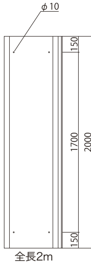
■断面図 寸法単位 (mm)
