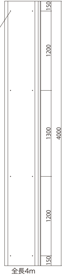
■立面図 寸法単位 (mm)
